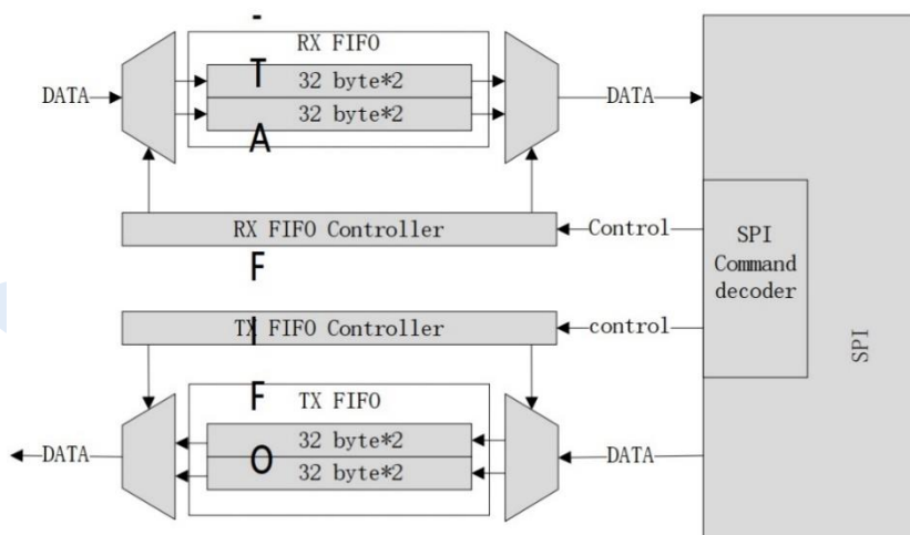
FIFO 框图
